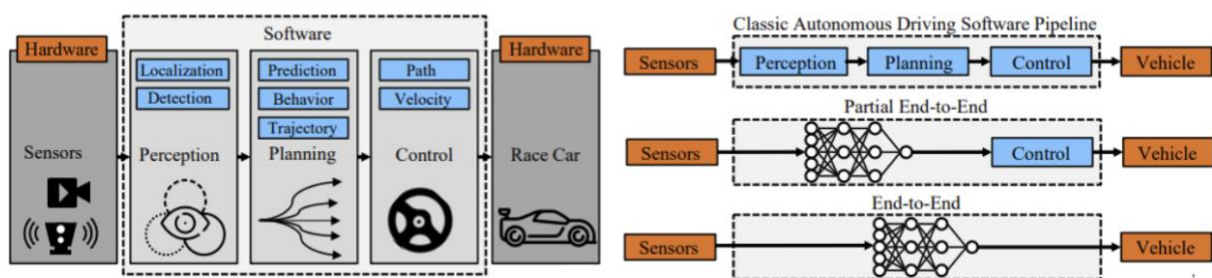
Figure 3 : a) Exemple d'une solution Edge IA pour véhicule autonome ; b) Analyse des différences entre le pipeline logiciel traditionnel de conduite autonome et les pipelines logiciels complets et partiels. [14]
